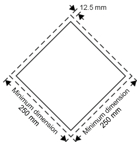
Figur 5.3.1.7.1: Storetikett (utom för klass 7)
