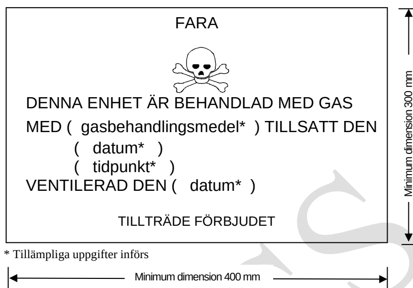
Figur 5.5.2.3.2: Varningsmärkning för gasbehandlad lastbärare
