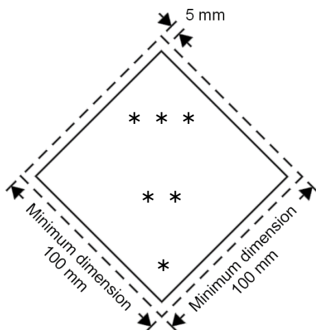
Figur 5.2.2.2.1.1: Etikett för klass
