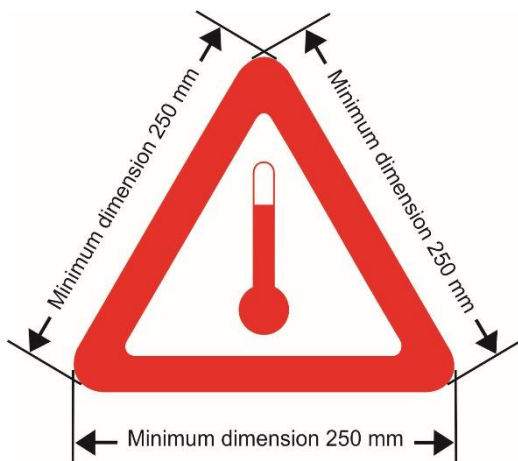
Figur 5.3.3: Märkning för ämnen som transporteras vid förhöjd temperatur
