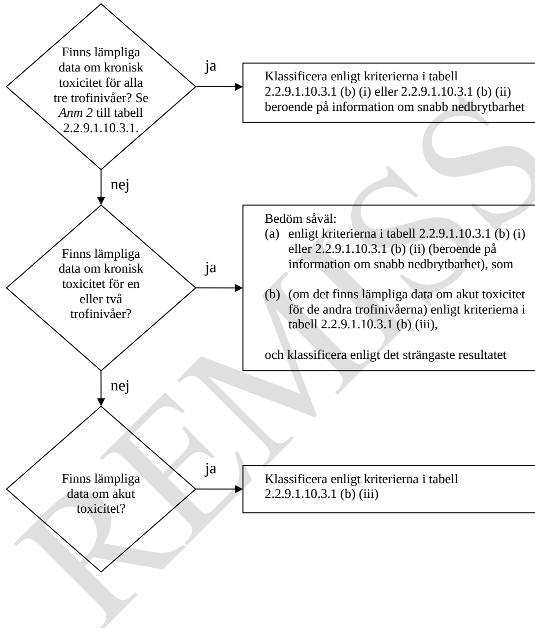
Figur 2.2.9.1.10.3.1: Kategorier för ämnen som har skadliga långtidseffekter för vattenmiljön
